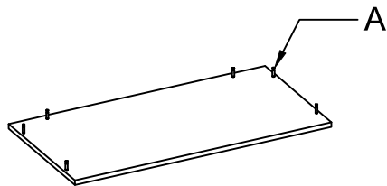
Top plate :800x400x25=1
