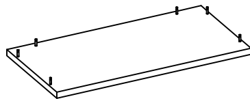
bottom plate :800x400x25=1
